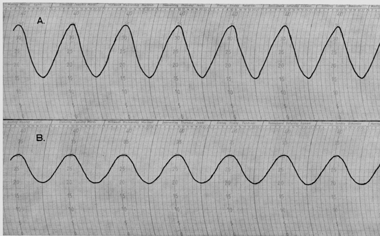
FIG. 1. — Allure des variations thermiques dans les traitements à température fluctuante. A: 15-35°C; B: 20-30°C.
