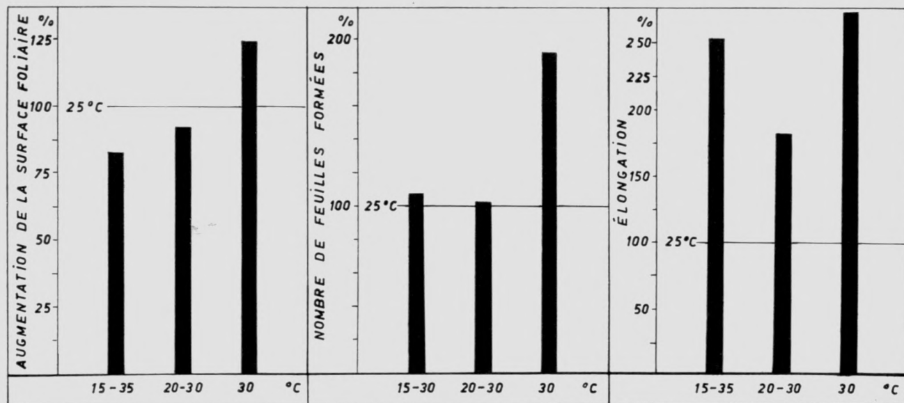
FIG. 7. — Quelques paramètres de la croissance du cacaoyer pour les divers traitements thermiques (en % du témoin maintenu à 25°C). Les valeurs indiquées représentent une moyenne des essais 4, 5 et 6.
