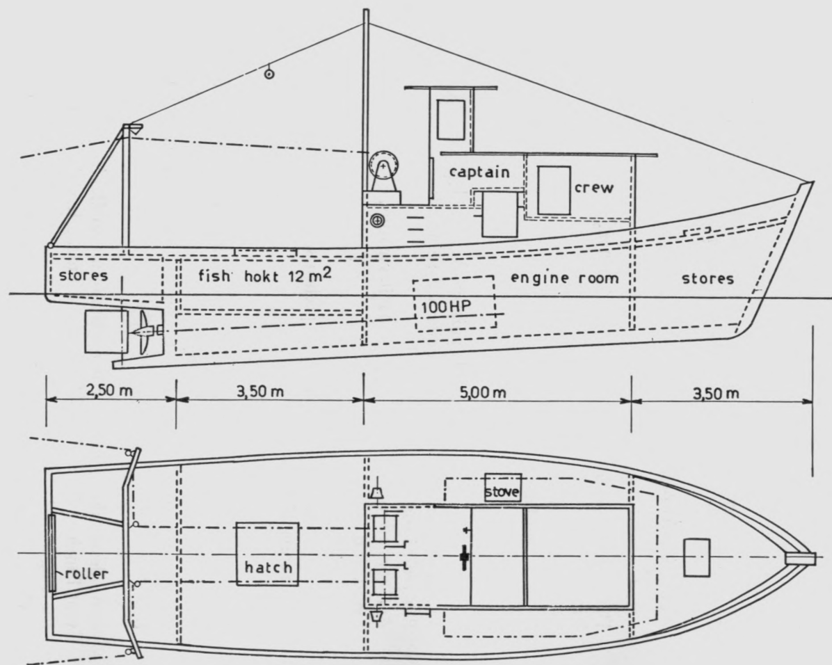
Fig. 4 — Chalutier pêcheant par l'arrière.
