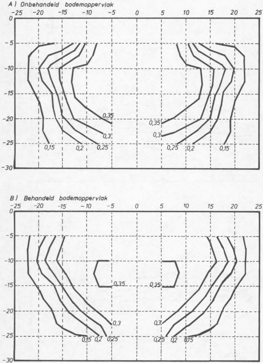
Fig. 14. — Vergelijking bij een vochtinfiltratieproef waarbij de bodemoppervlakte in het ene geval niet en in het andere geval wel werd behandeld met een bitumen-emulsie. Bemerkt het hogere vochtgehalte in dit laatste geval tot vlak bij het oppervlak in de bovenste 20 cm.
