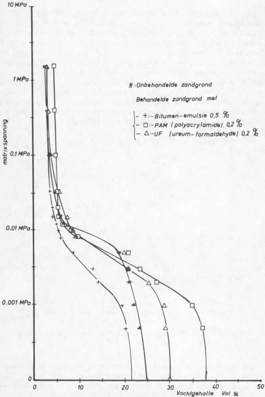
Fig. 3. — Verband tussen de hoeveelheid gebonden water en de zuigspanning waarmede het in een woestijnzandgrond wordt vastgehouden. Bemerk de invloed van een bitumen behandeling waarbij het vocht minder hard wordt vastgehouden (hydrofoob), en van de andere behandelingen die het water meer vasthouden (hydrofiel) dan in het oorspronkelijke monster.
