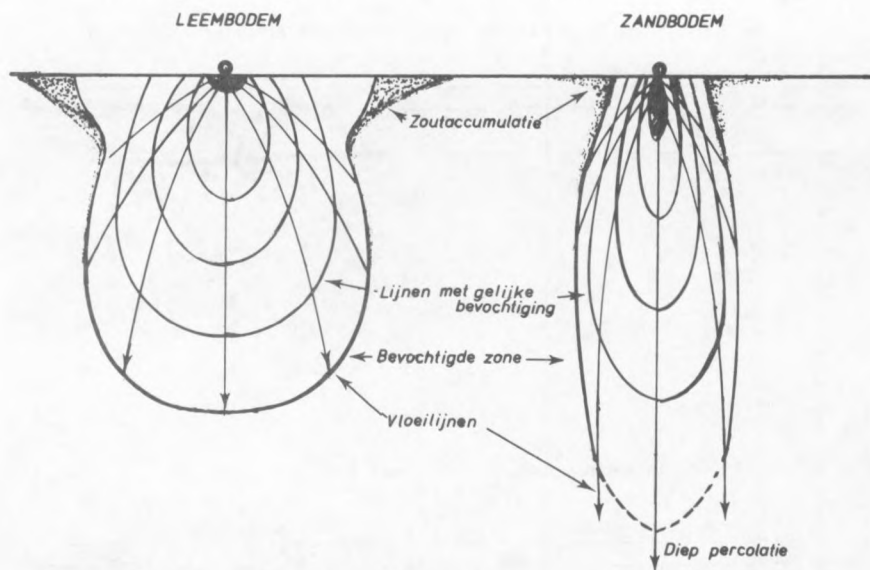
Fig. 8. — Bevochtigingsprofiel in de bodem vanuit een dripopening ; links een leemhoudende grond, rechts een zandbodem. In het laatste geval is de verticale component dominerend en treedt groot waterverlies op door diep percolatie. Links blijft het water dicht bij de oppervlakte, er heeft veel verdamping plaats, wat bodemverzilting tot gevolg heeft.
