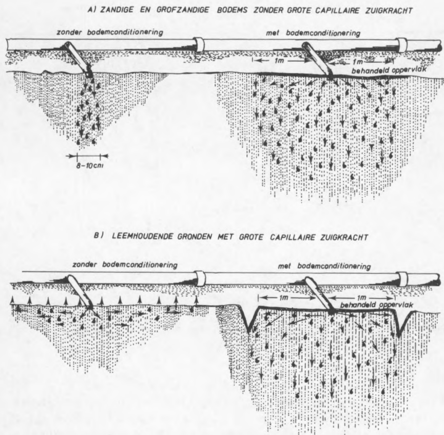
Fig. 7. — Bevochtigingsprofiel bij druppelirrigatie naargelang de grondsoort en het al dan niet toedienen van een hydrofoob bodemkonditioneringsmiddel aan de oppervlakte. Dank zij dit laatste kan men zowel in een zandige als in een lemige bodem een homogene spreiding van de ganse wortelzone bekomen en meteen het waterverlies tegengaan.
