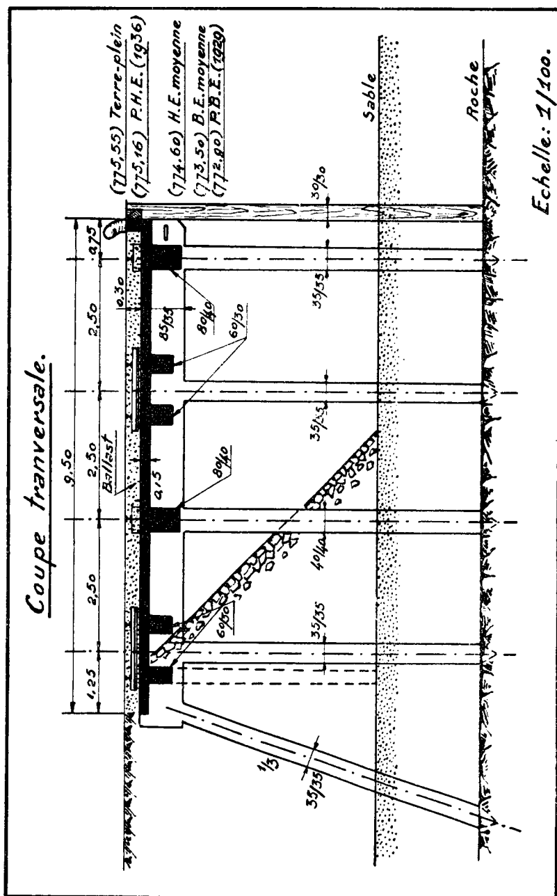
Fig. 22. — Appontement d'Albertville (coupe transversale).
