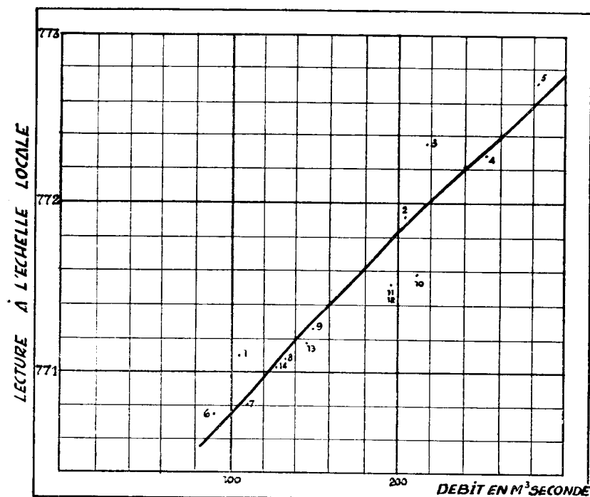
FIG. 11. — Débits de la Lukuga à Greinerville.
