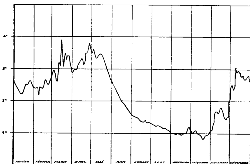
FIG. 13. — Variations journalières du niveau du Lualaba (Bief moyen) à Kindu en 1946.
