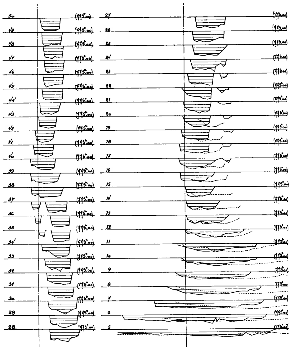
Variations des profils en travers de l'exutoire de la Lukuga de juin 1937 à février 1941, depuis la traverse 5 jusqu'à la traverse 50 (voir Planche I).
