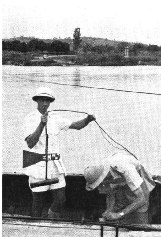
PHOTO 10. — Jaugeage de la Lukuga. Mesure des vitesses de courant par moulinet Salmoiraghi. 9 septembre 1947.
