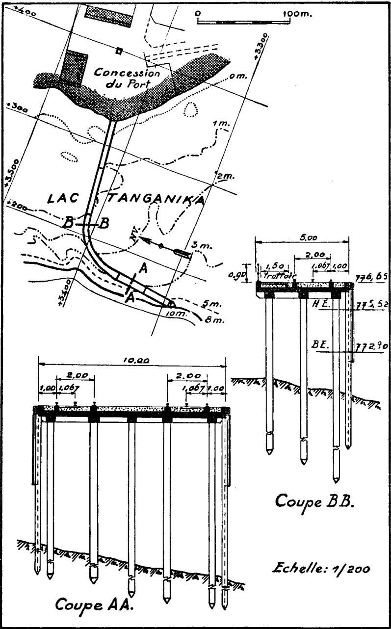
FIG. 25. — Situation et appontement du port d'Usumbura
