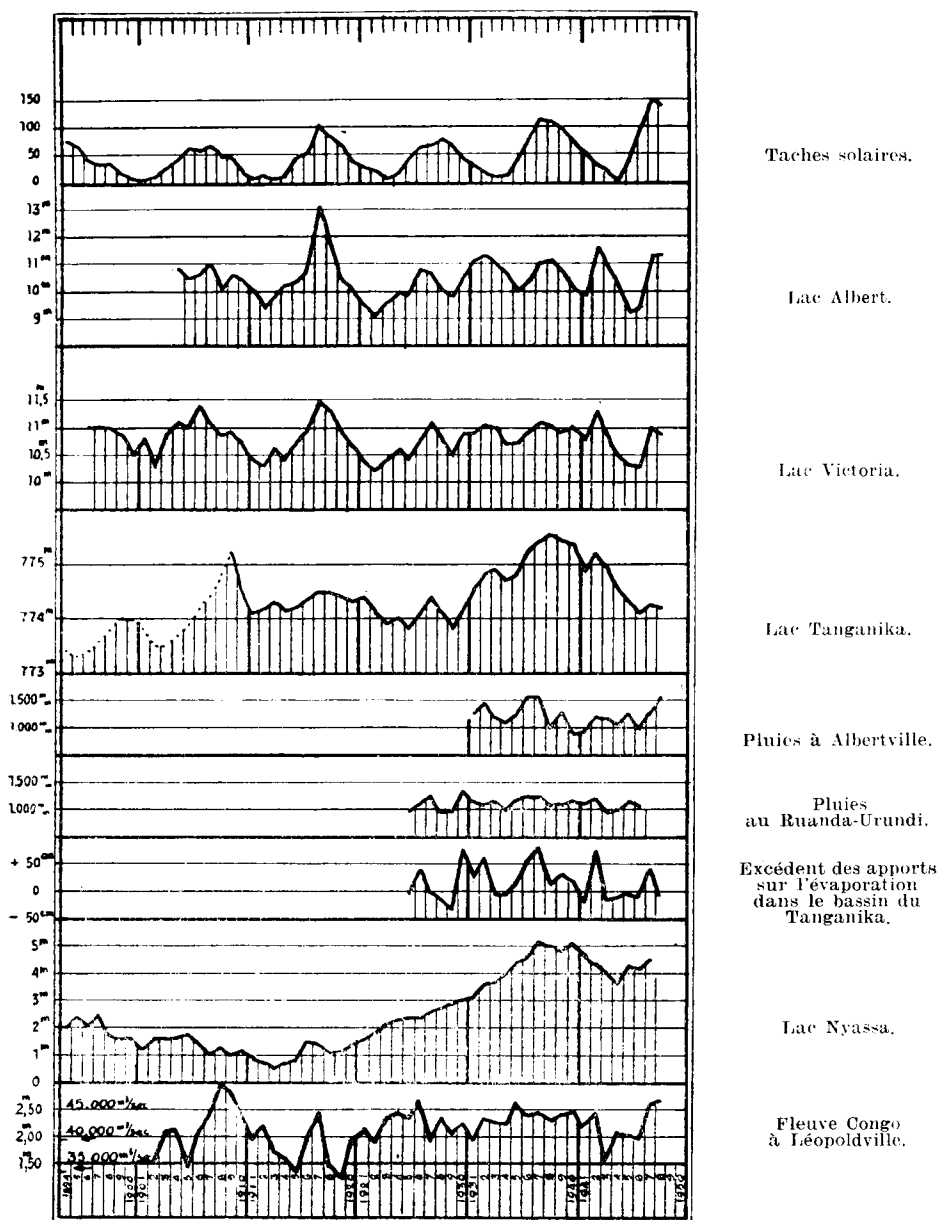
FIG. 7. — Taches solaires.
