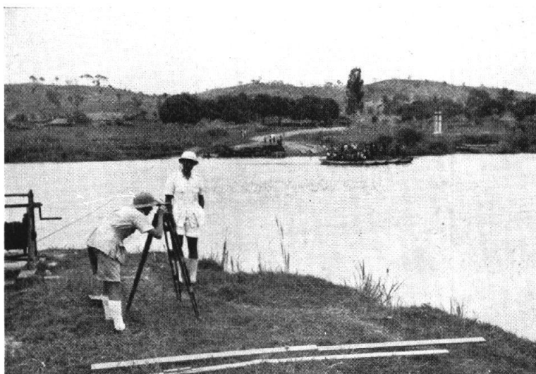
PHOTO 9. — La Lukuga au passage du bac à traîlle de la route automobile Albertville-5 e parallèle; à gauche, le treuil du câble de jaugeage. 9 septembre 1947.
